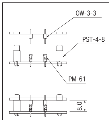
二段重ね用端子と使用した状態
