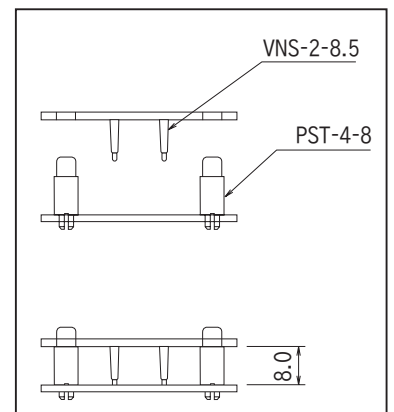
スプリングプローブと使用した状態
